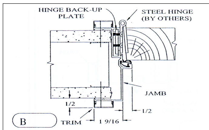
HINGE JAMB
