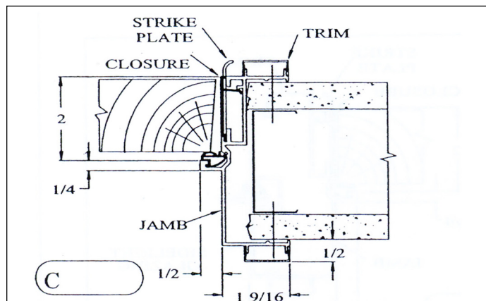
STRIKE JAMB
